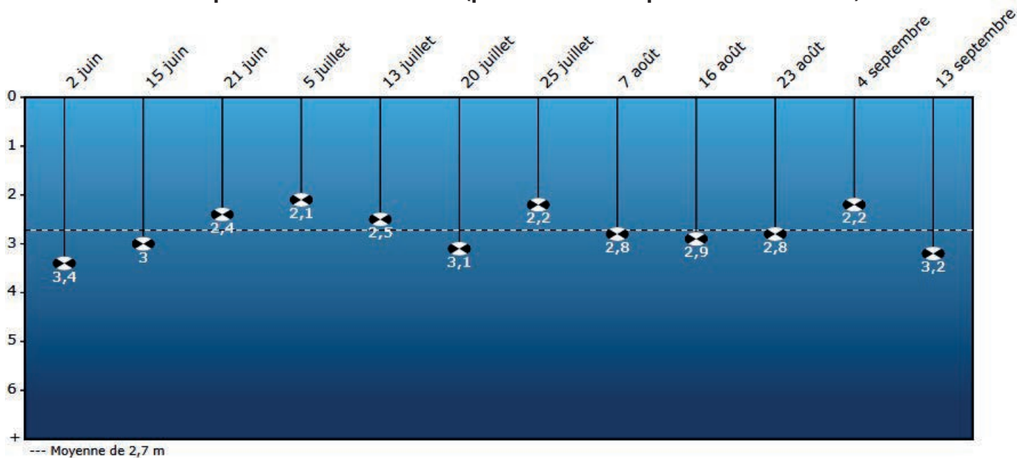
Transparence de l'eau - Été 2021 (profondeur du disque de Secchi en mètre)
